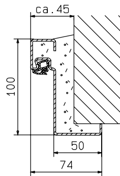
Zarge "ZG 68/76" (begrenzter Maßbereich)
