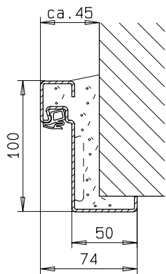
Hauptzarge "ZG/ZNG 68/76"
